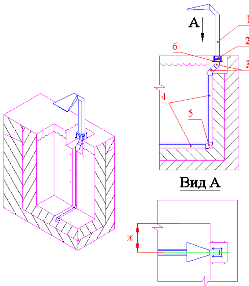
Рисунок 5 (скиммерной бассейн) (прокладка трубопроводов по дну бассейна)
